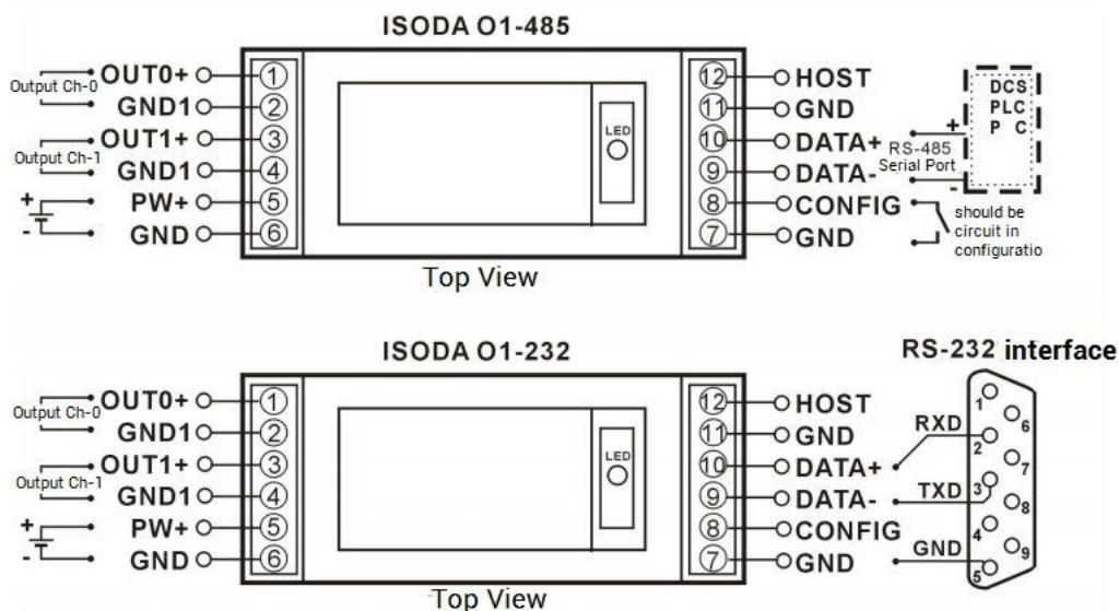
Fig. 3 ISODA module wiring scheme
